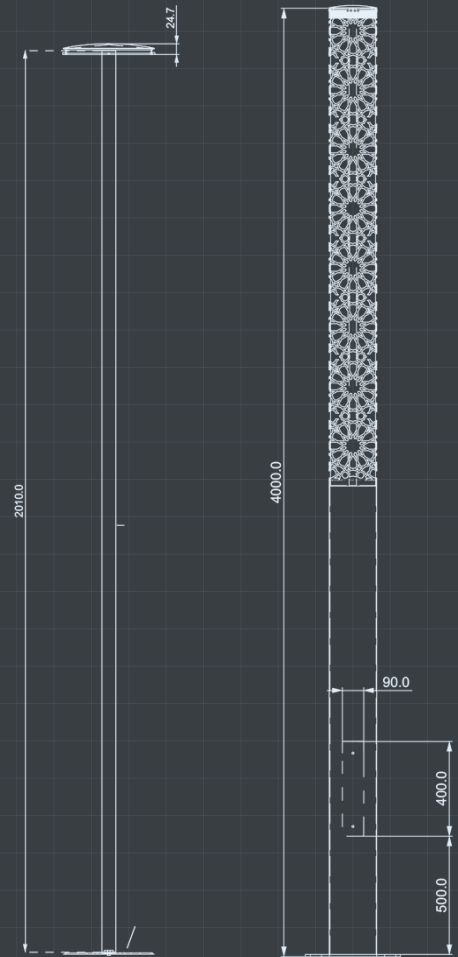
وحدة 1 950 + غطاء - جذع العمود 2 000 مم قطع مركزي ألومنيوم 20 × 20 × L 2 010
