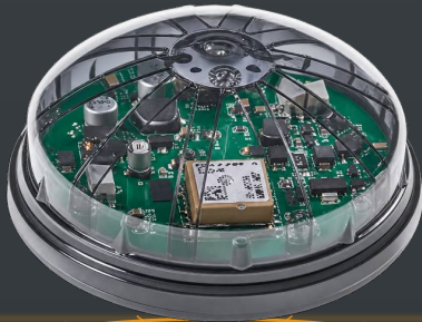
عقدة LiDAR من D-SLS على قاعدة D4i — Zhaga Book 18 • 20، قابل للتثبيت بالمشبك في أي وقت دون فتح العمود
